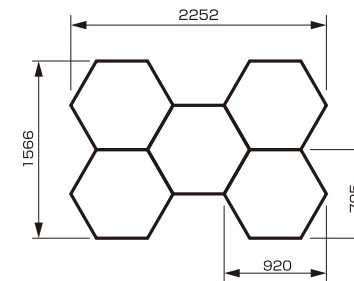
1セット組立サイズ(一例)
