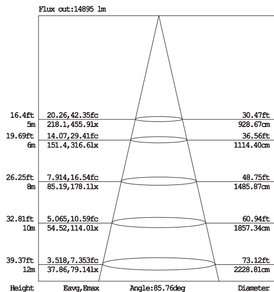
照度図
