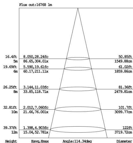
照度図
