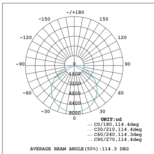
配光曲線
