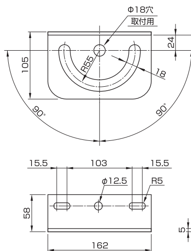
アダプター外形寸法図
