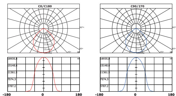
配光曲線
