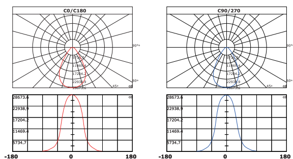
配光曲線
