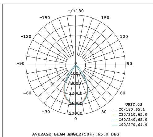
配光曲線
