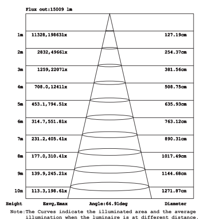
照度図
